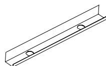
FESTER KABELKANAL FÜR GERADE THEKEN
